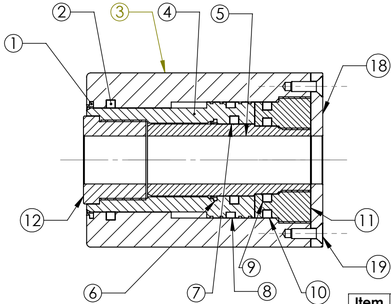
SECTION A-A SCALE 1 : 3
